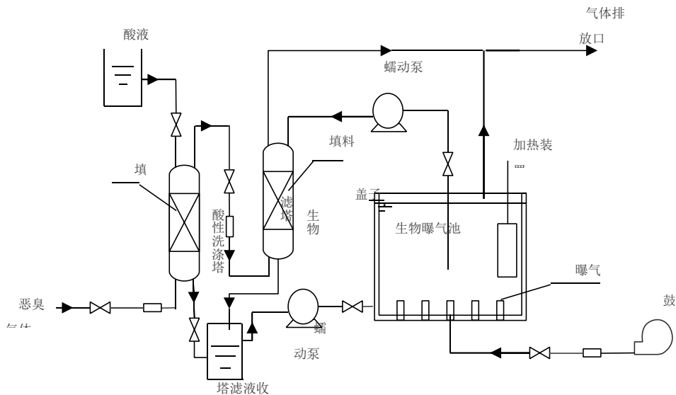
图 6-3 恶臭气体处理工艺流程图
