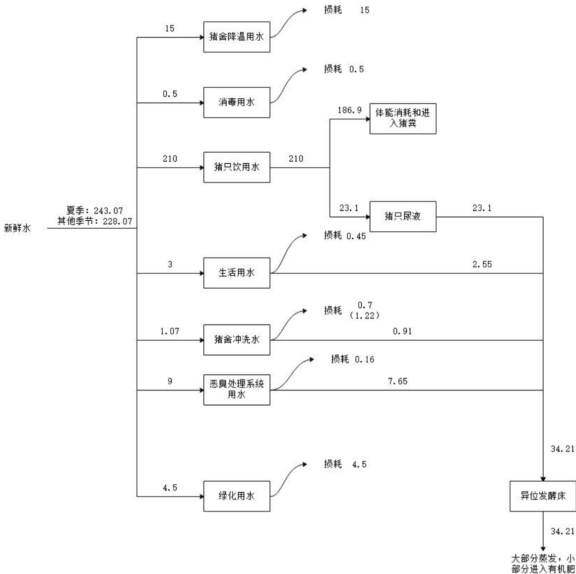
图 3-6 项目水平衡图 单位 m³/d
