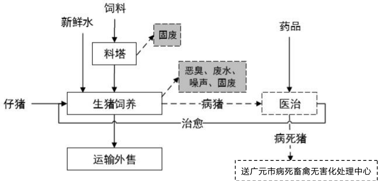
图 3-2 项目养殖工艺流程及产污位置图
